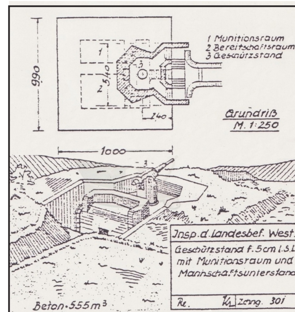
Plan d'époque d'une casemate R 600
